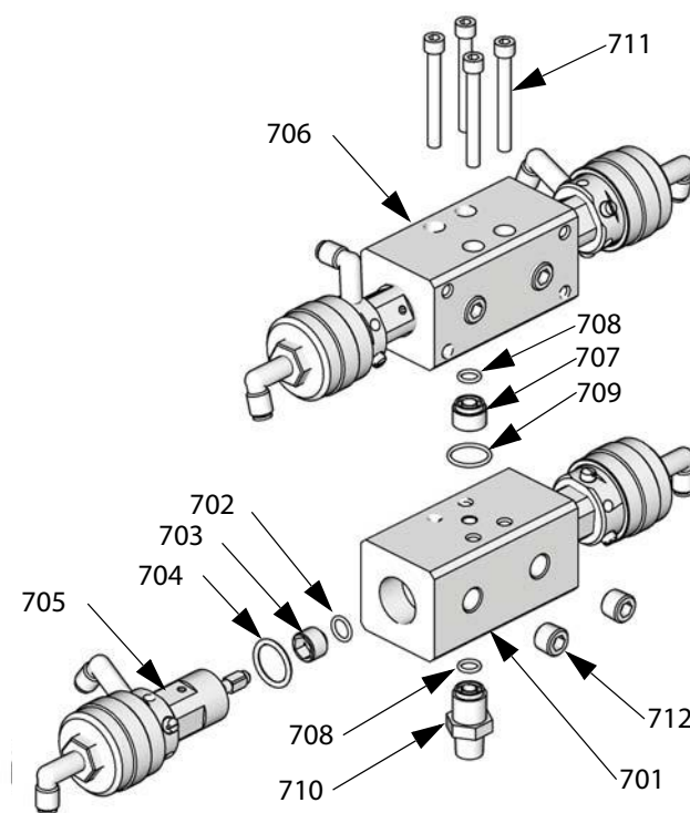
Рис. 23. Повторная установка дозирующих клапанных блоков
