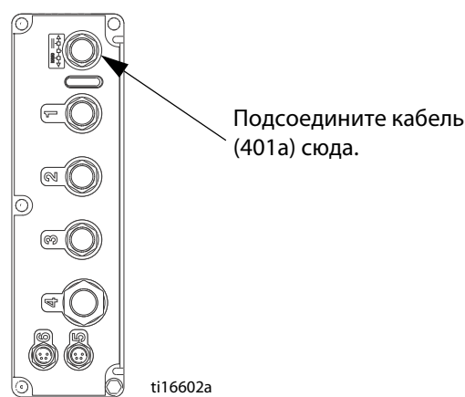
Рис. 6. Снова подключите CAN-кабель.
