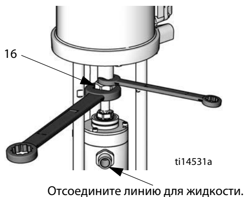
Рис. 26. Ослабление стяжной муфты
