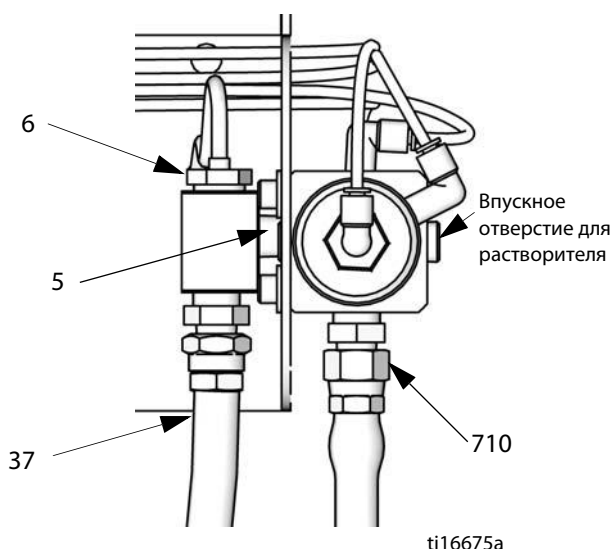
Рис. 21. Отсоединение линии для жидкости
