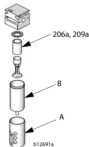
Рис. 2. Замена элемента(ов) воздушного фильтра
