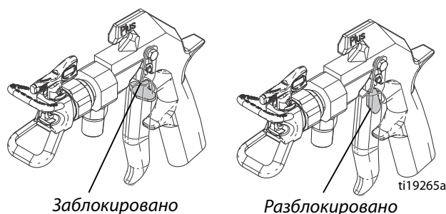
Рис. 1. Положения блокиратора пускового курка
