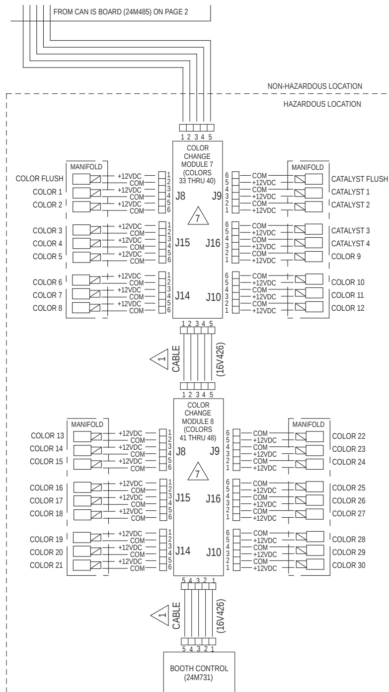
Figure 29 Электросхема, лист 3, опасная зона
