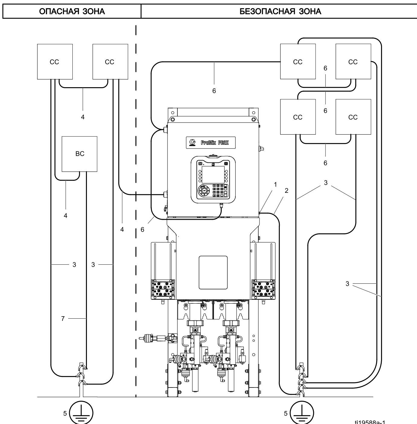
Figure 23 Заземление системы
