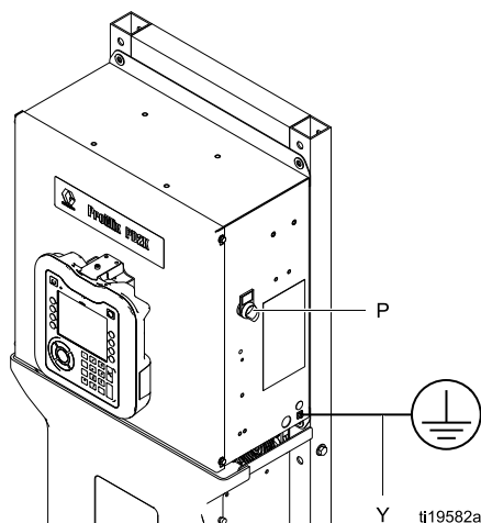
Figure 22 Винт заземления и выключатель питания
