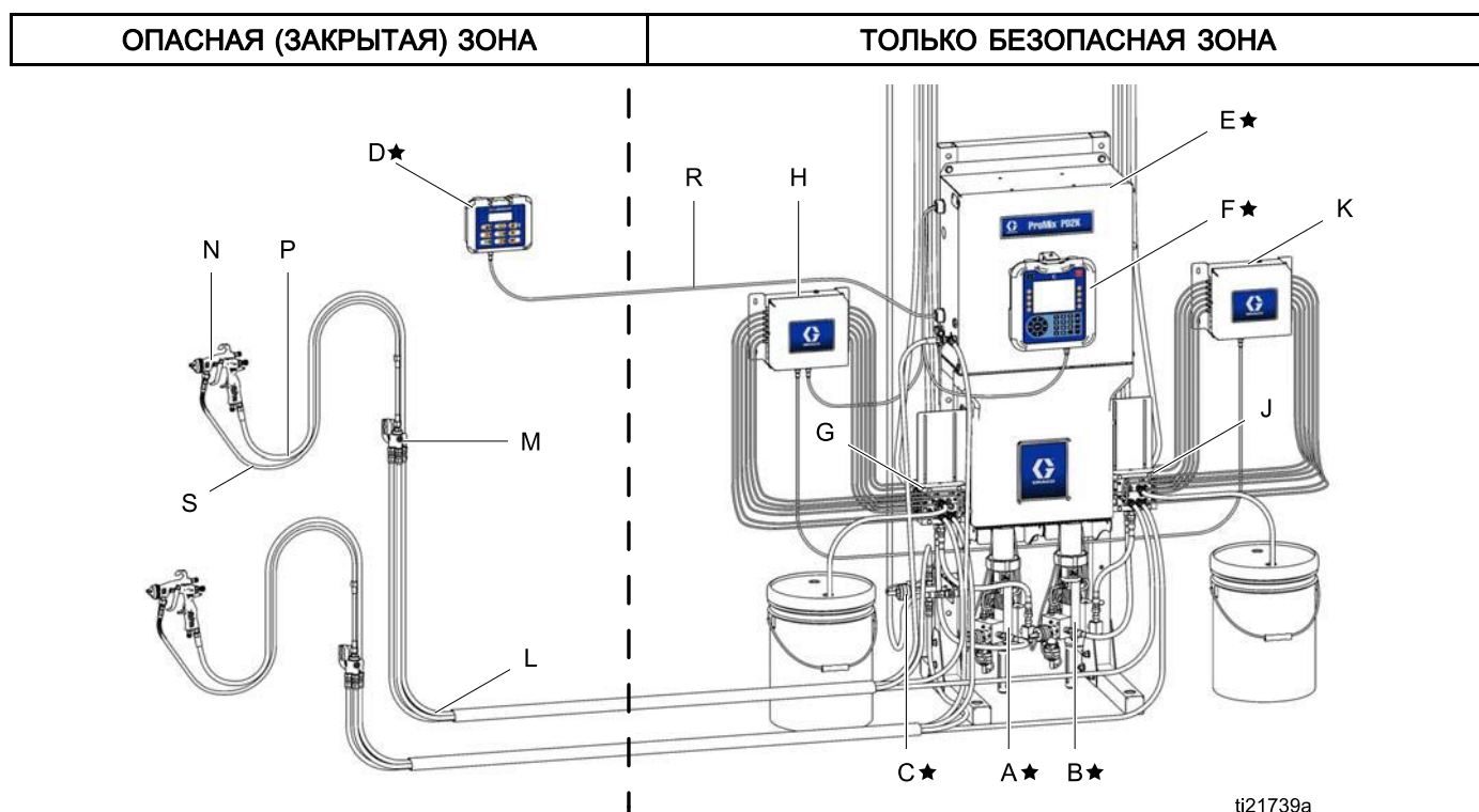
Figure 9 Типовая установка
