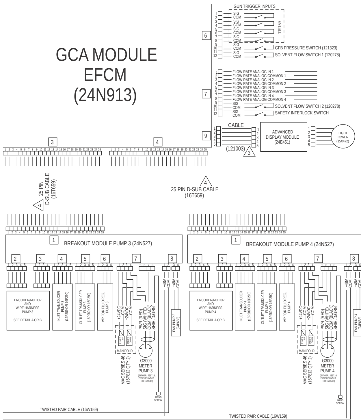
Figure 26 Электросхема, лист 2, часть 2 ПРОДОЛЖЕНИЕ НА СЛЕДУЮЩЕЙ СТРАНИЦЕ
