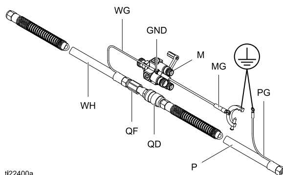
Figure 20 Комплект быстроразъемного соединения для электростатического клапана подачи воздуха
