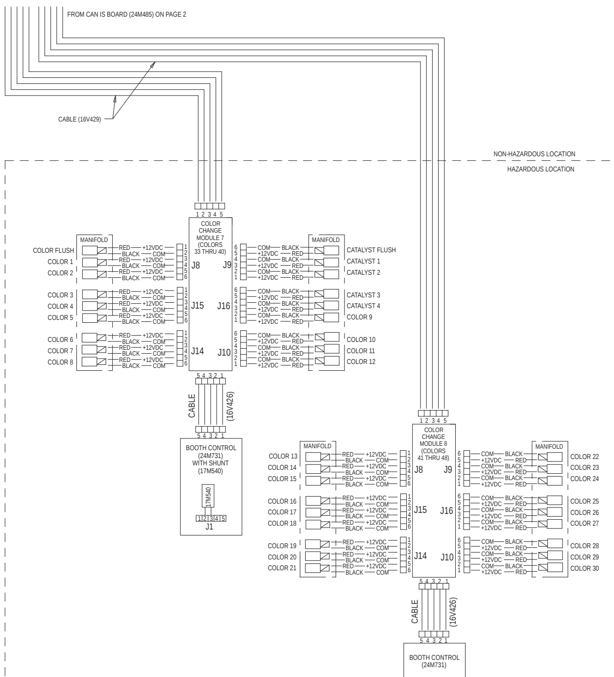
Figure 34 Электросхема, лист 3, часть 2
