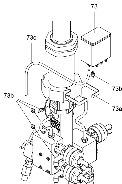
Figure 19 Установка комплекта крышек для жидкости щелевых уплотнений
