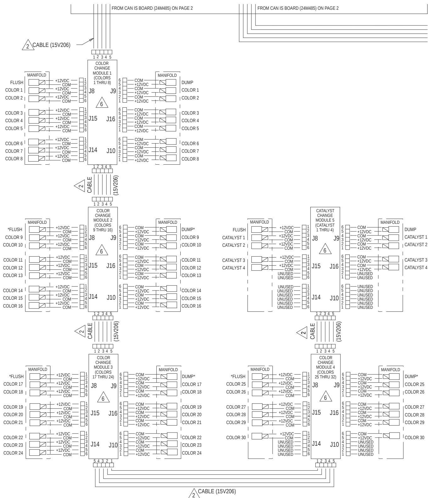
Figure 27 Электросхема, лист 3
