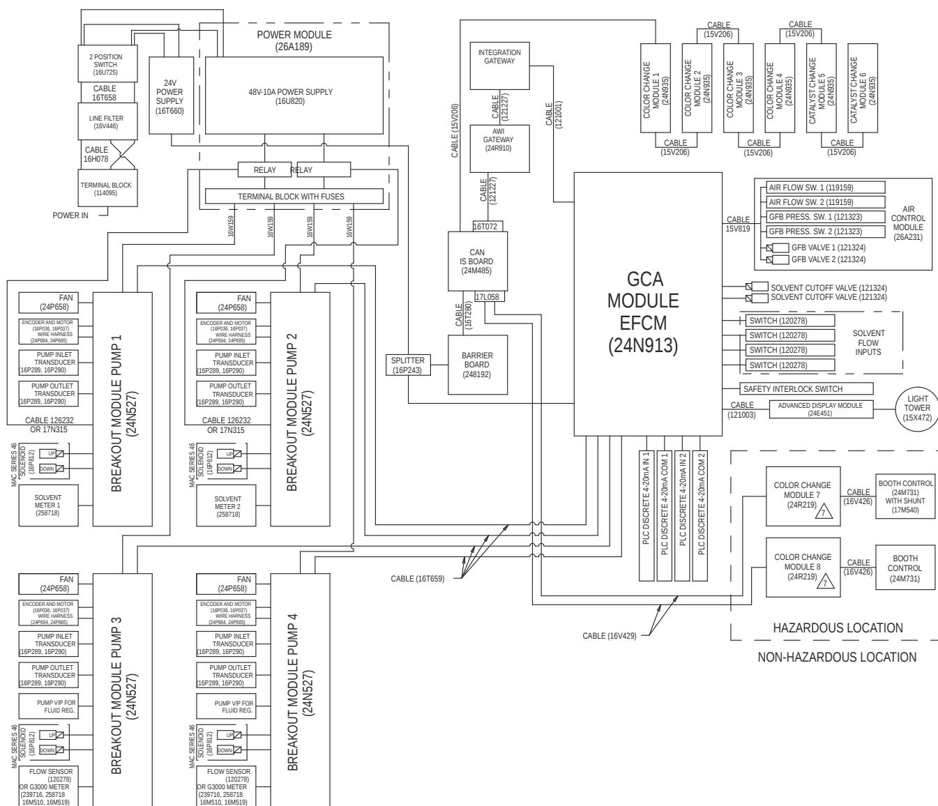
Figure 30 Электросхема, лист 1
