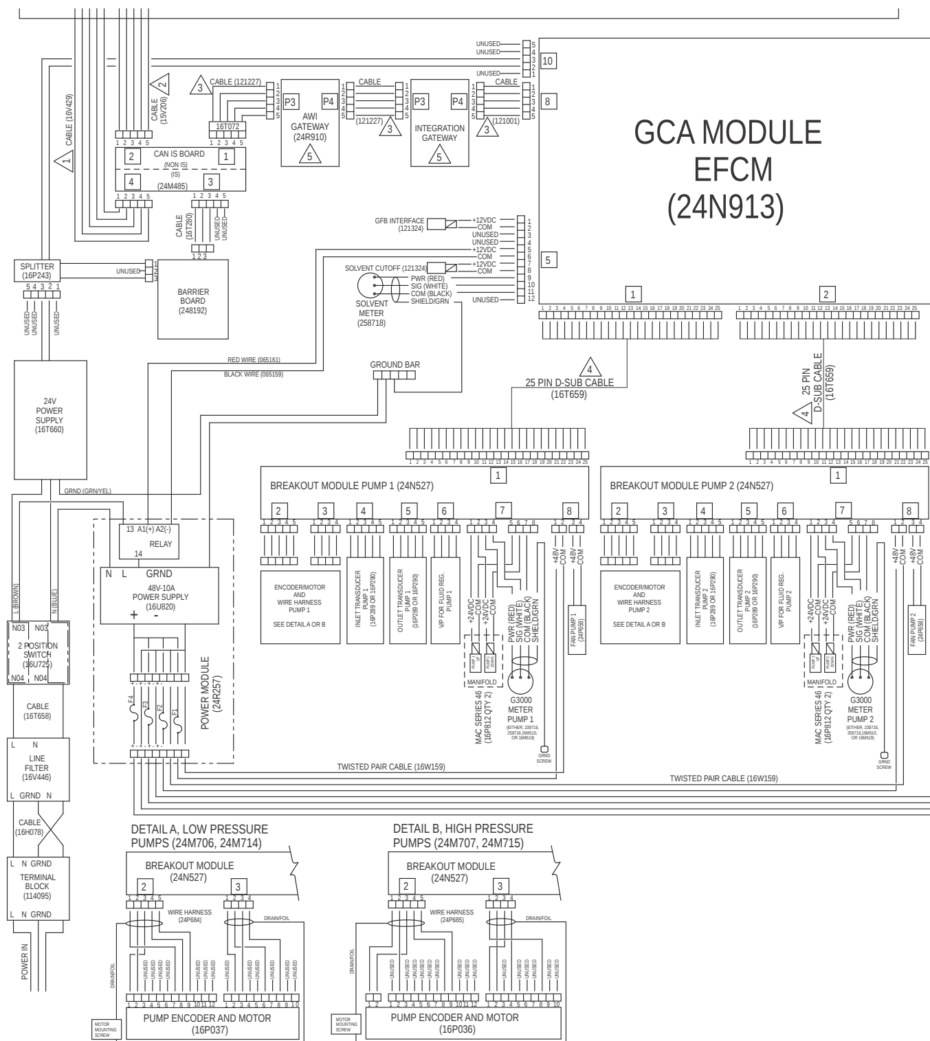
Figure 25 Электросхема, лист 2, часть 1 ПРОДОЛЖЕНИЕ НА СЛЕДУЮЩЕЙ СТРАНИЦЕ
