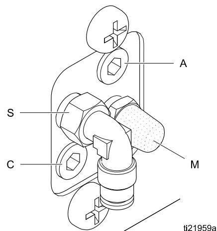
Figure 17 Соединения воздушного коллектора Обозначения
