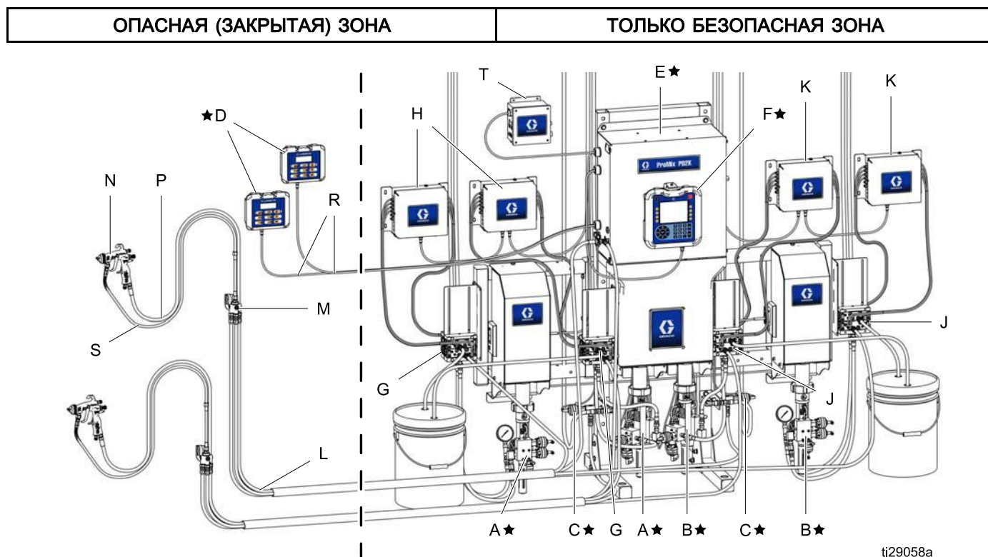
Figure 11 Типовая установка с двумя панелями (MC1002, MC2002, MC4002)
