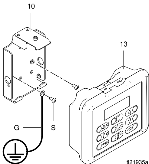
Figure 14 Заземление кронштейна устройства управления окрасочной камерой
