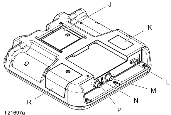
Figure 13 Соединительные порты расширенного модуля дисплея
