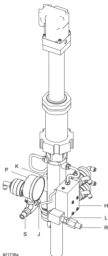
Figure 18 Впускные и выпускные соединения насоса
