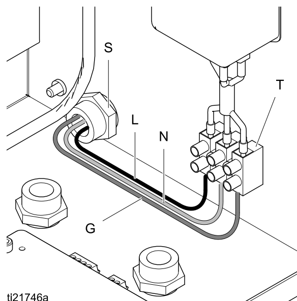
Figure 21 Электрическое соединение блока управления
