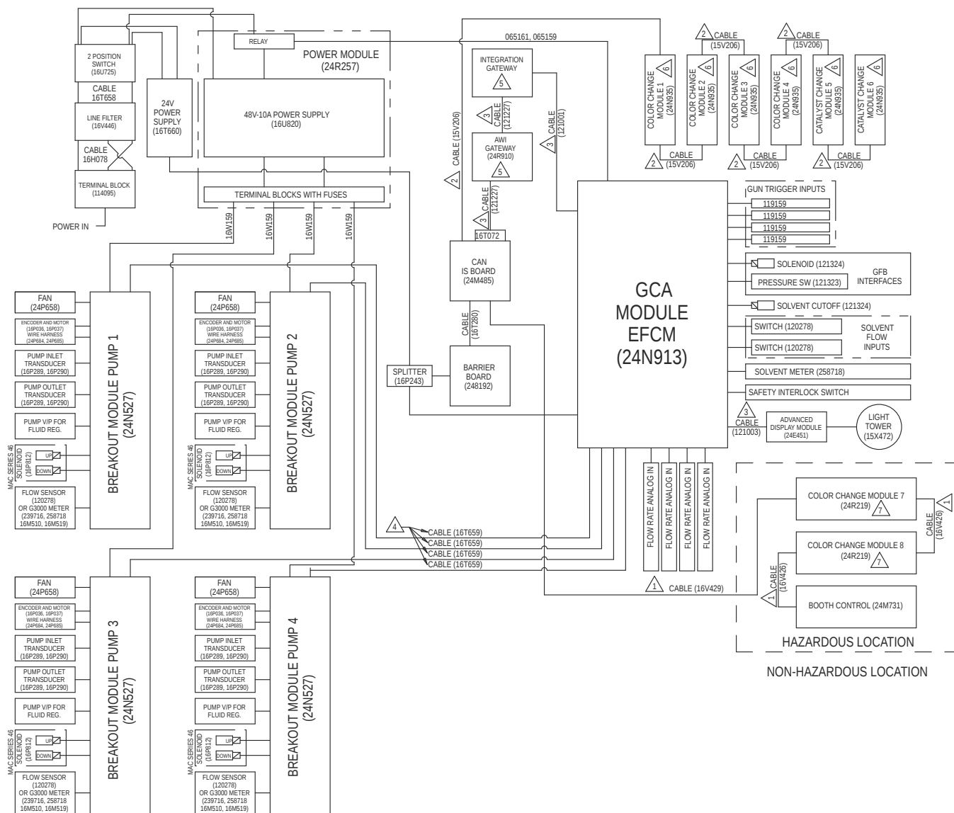
Figure 24 Электросхема, лист 1
