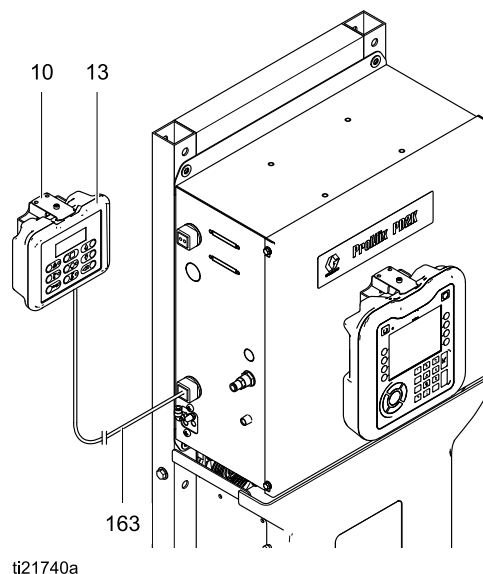
Figure 15 Установка устройства управления окрасочной камерой
