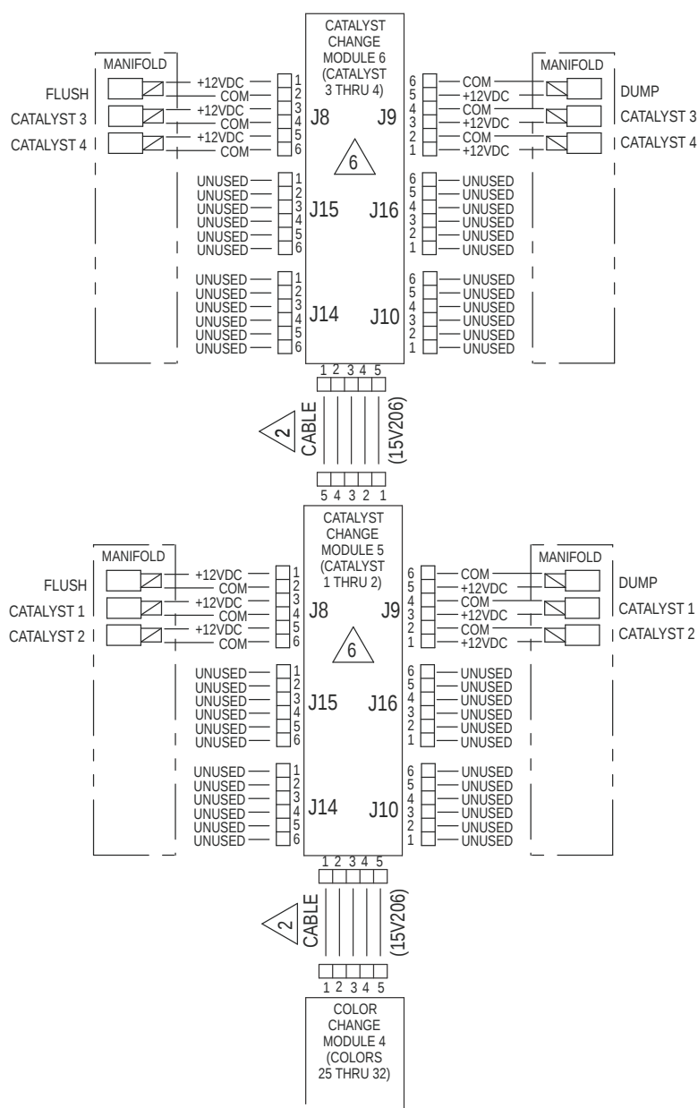
Figure 28 Электросхема, лист 3, дополнительная конфигурация для устройства управления сменой катализатора
