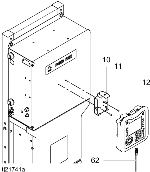
Figure 12 Установка модуля дисплея
