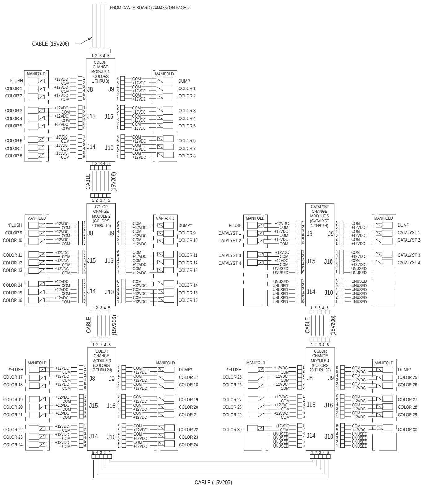
Figure 33 Электросхема, лист 3, часть 1
