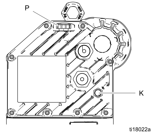
Figure 5 Смотровое стекло и крышка маслозаливного отверстия
