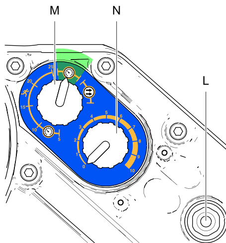
Figure 11 Режим контроля давления
