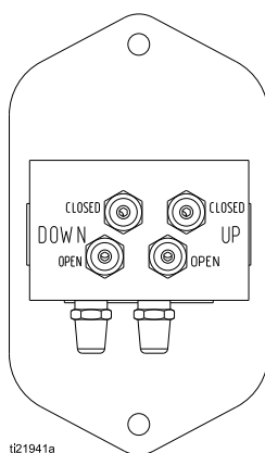
Figure 4 Трубные соединения соленоидного коллектора с коллектором на впуске насоса
