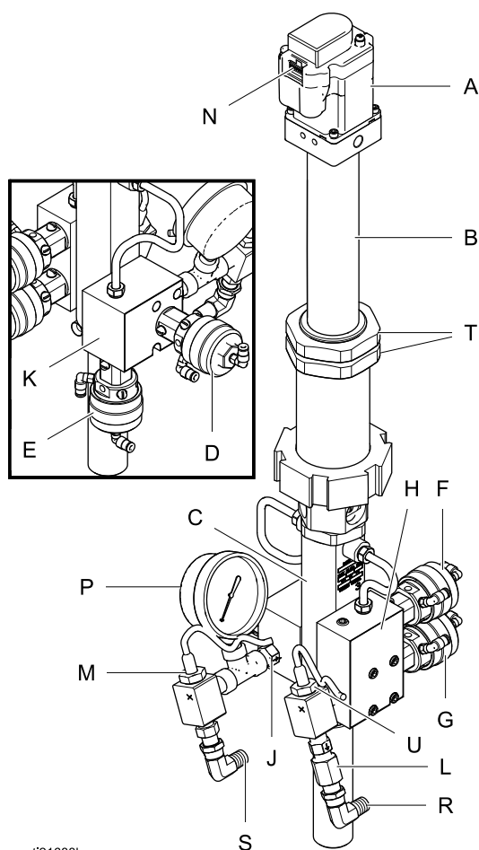
Figure 3 Компоненты насоса
