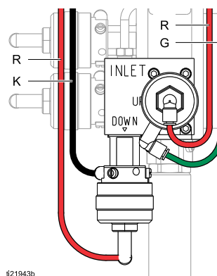
Figure 5 Соединения трубопровода впускного коллектора
