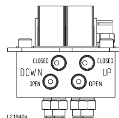
Figure 6 Трубные соединения соленоидного коллектора с коллектором на выпуске насоса
