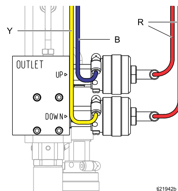
Figure 7 Соединения трубопровода выпускного коллектора
