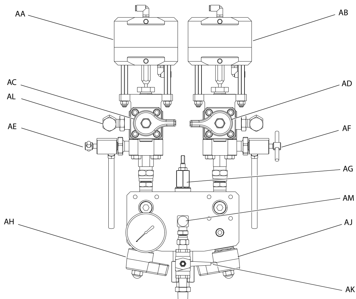
Рис. 3: Блок управления подачей материала
