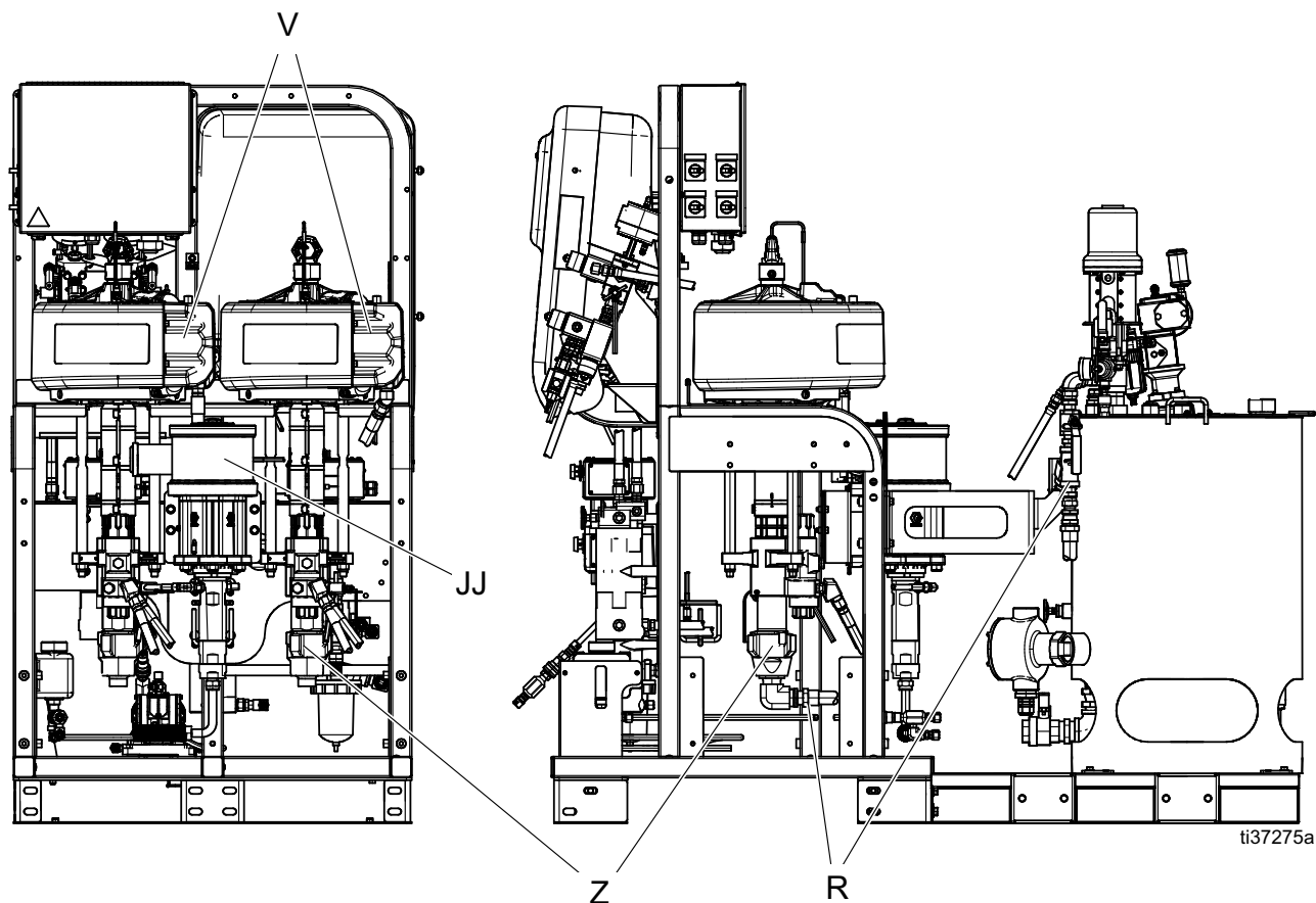
Рис. 2: Типовая установка: Бункер с двойными стенками на 95 литров с рециркуляцией (вид сзади и сбоку)
