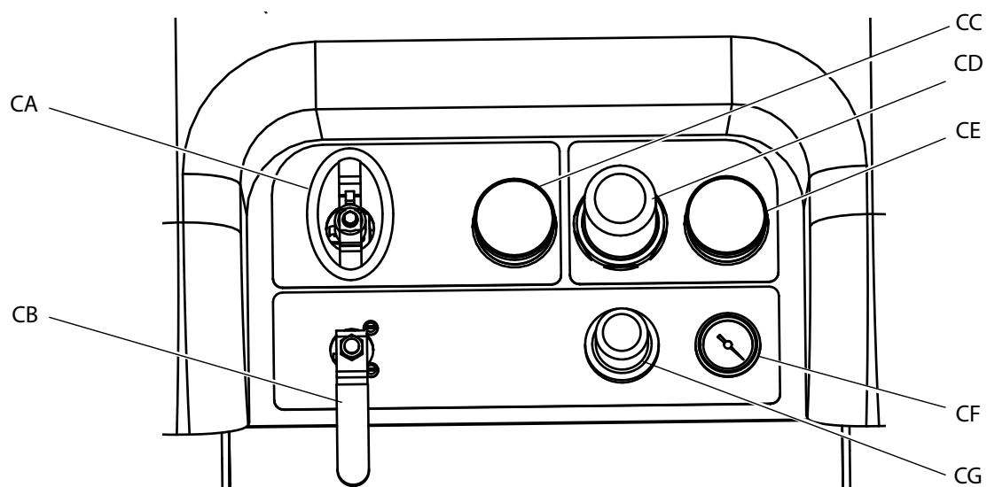
Рис. 4: Пневмоклапаны
