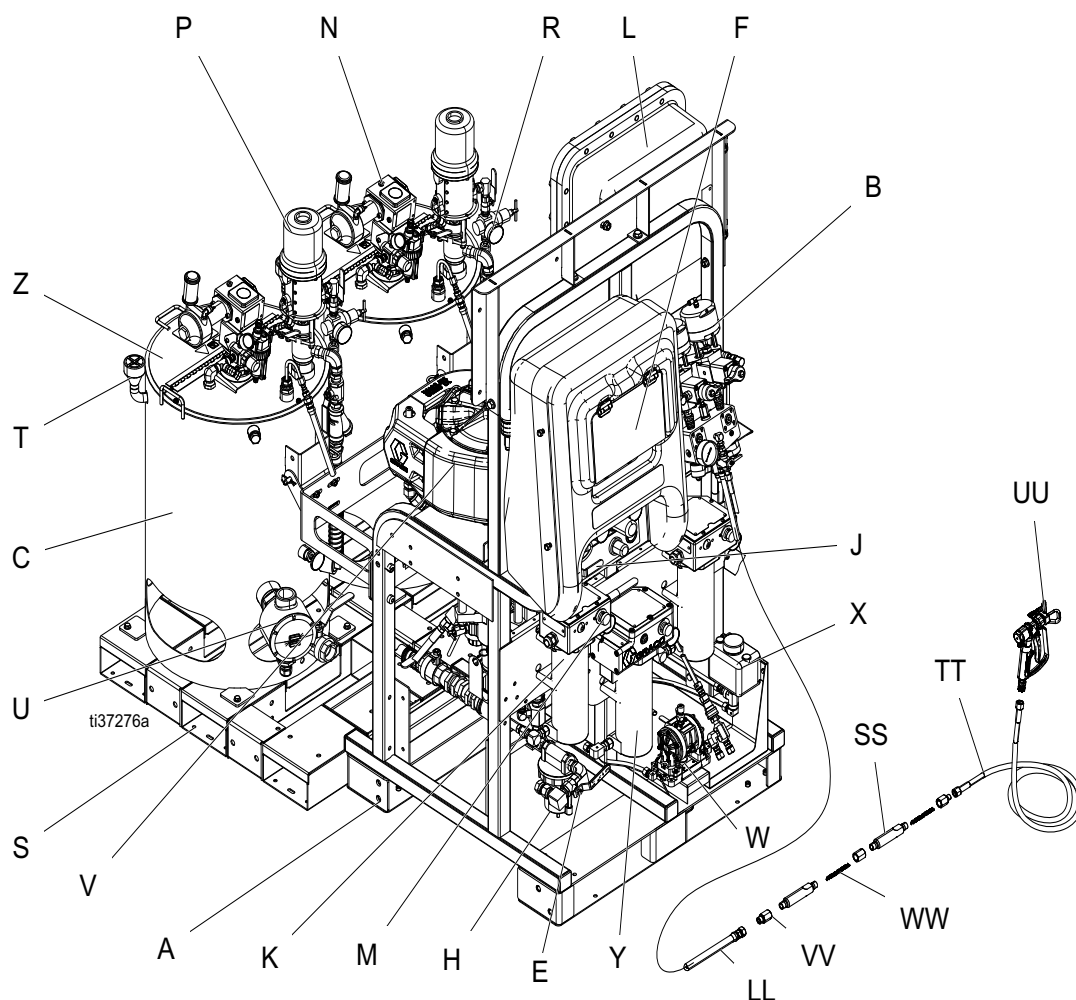
Рис. 1: Типовая установка: Бункеры объемом 95 литров с рециркуляцией (вид спереди)
