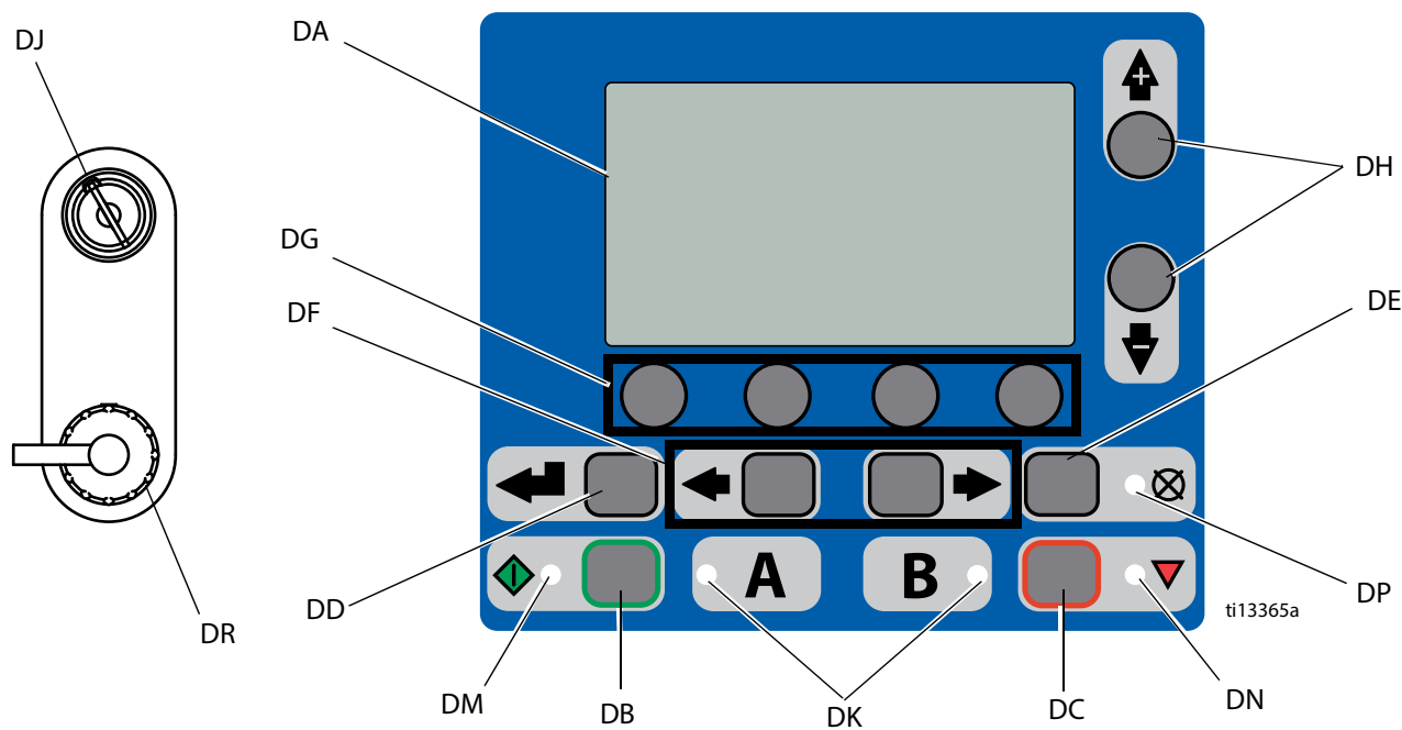
Рис. 5: Интерфейс пользователя
