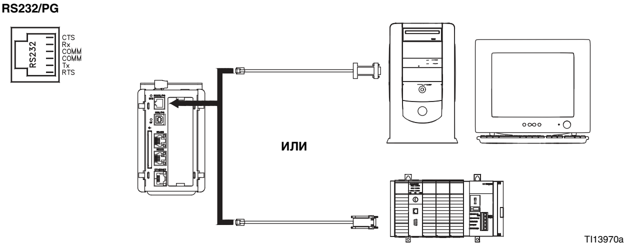
Рис. 8: Порты связи RS-232/PG
