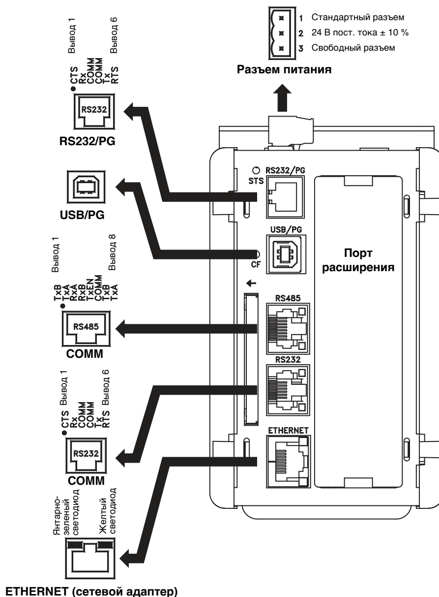
Рис. 5: Выводы портов Graco Gateway
