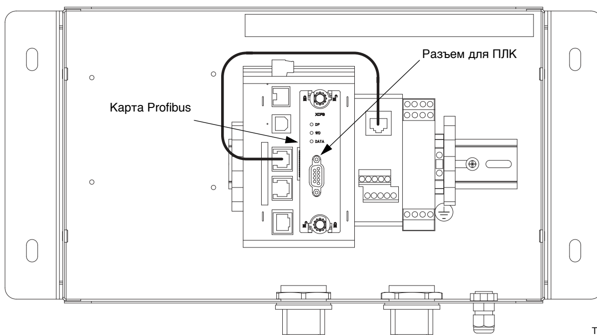
Рис. 48: Разъем для ПЛК Profibus
