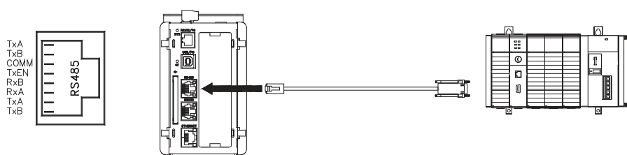
Рис. 6: Порт связи RS-485 (типовая схема подключения ProMix 2KS)
