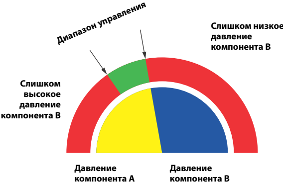
Рис. 50. Управляемый диапазон давления компонентов A/B при выборе ограничителя правильного размера
