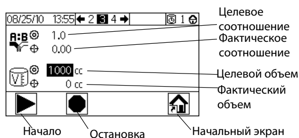
Рис. 28. Экран 3 (Смешивание: порция)
