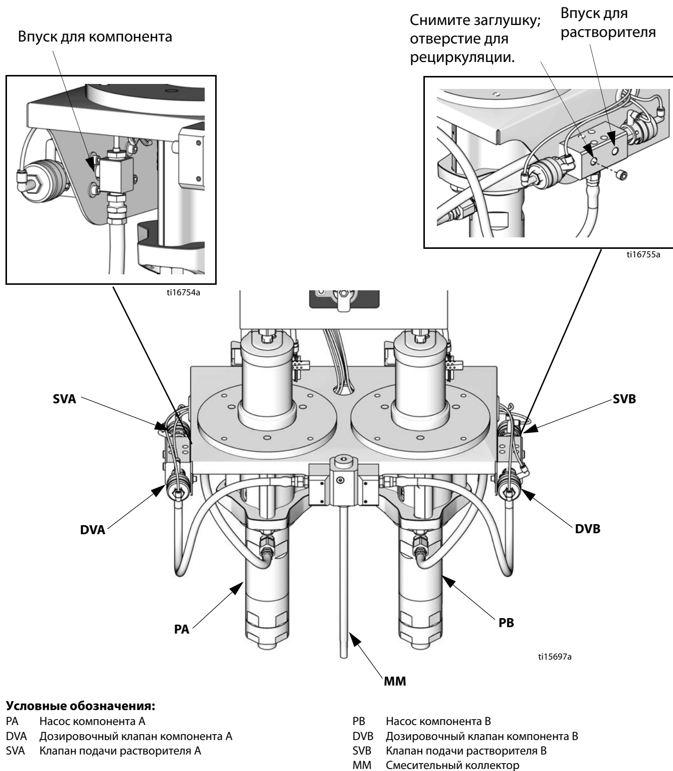
Рис. 5. Гидравлические соединения
