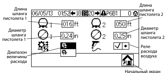
Рис. 38. Экран 19 (Настройка 2)
