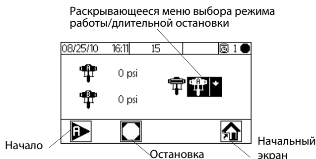
Рис. 33. Экран 15 (Управление насосом)
