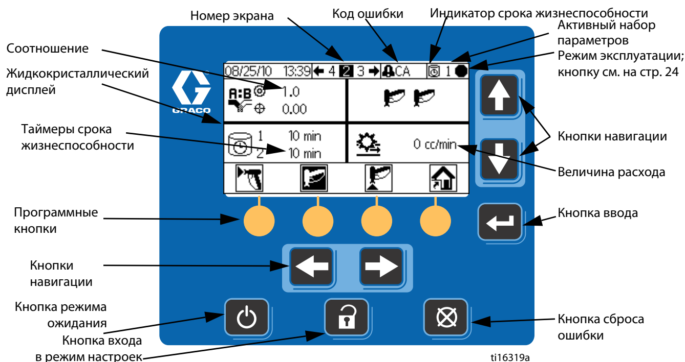
Рис. 10. Модуль дисплея
