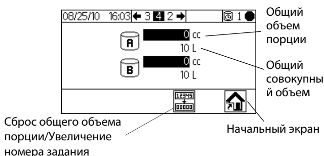
Рис. 29. Экран 4 (Смешивание: объемы)
