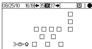
Рис. 47. Экран 36 (Тест мембраны)
