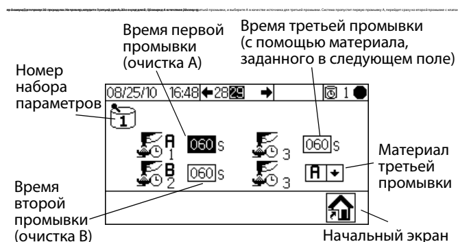
Рис. 41. Экран 29 (Набор параметров 1-2)
