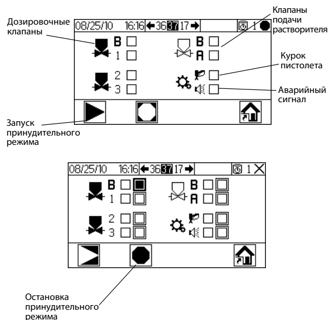
Рис. 48. Экран 37 (Поиск и устранение неисправностей: вывод данных на экран)
