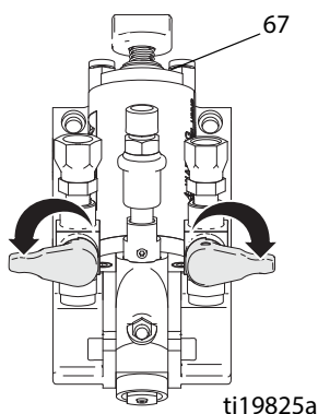
Рис. 13: Положение «закрыто» клапанов подачи материала
