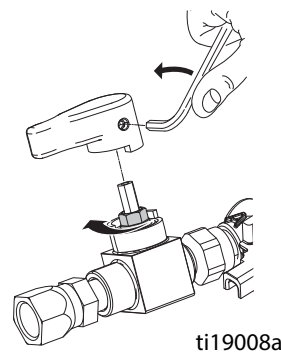
Рис. 10: Ослабьте уплотнительную гайку клапана подачи материала.
