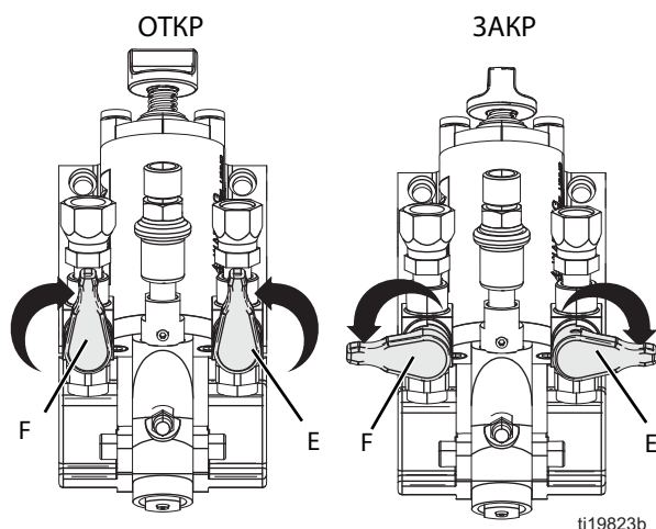
Рис. 5: Запорные клапаны
