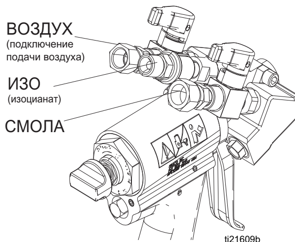
Рис. 2: Идентификация отверстия
