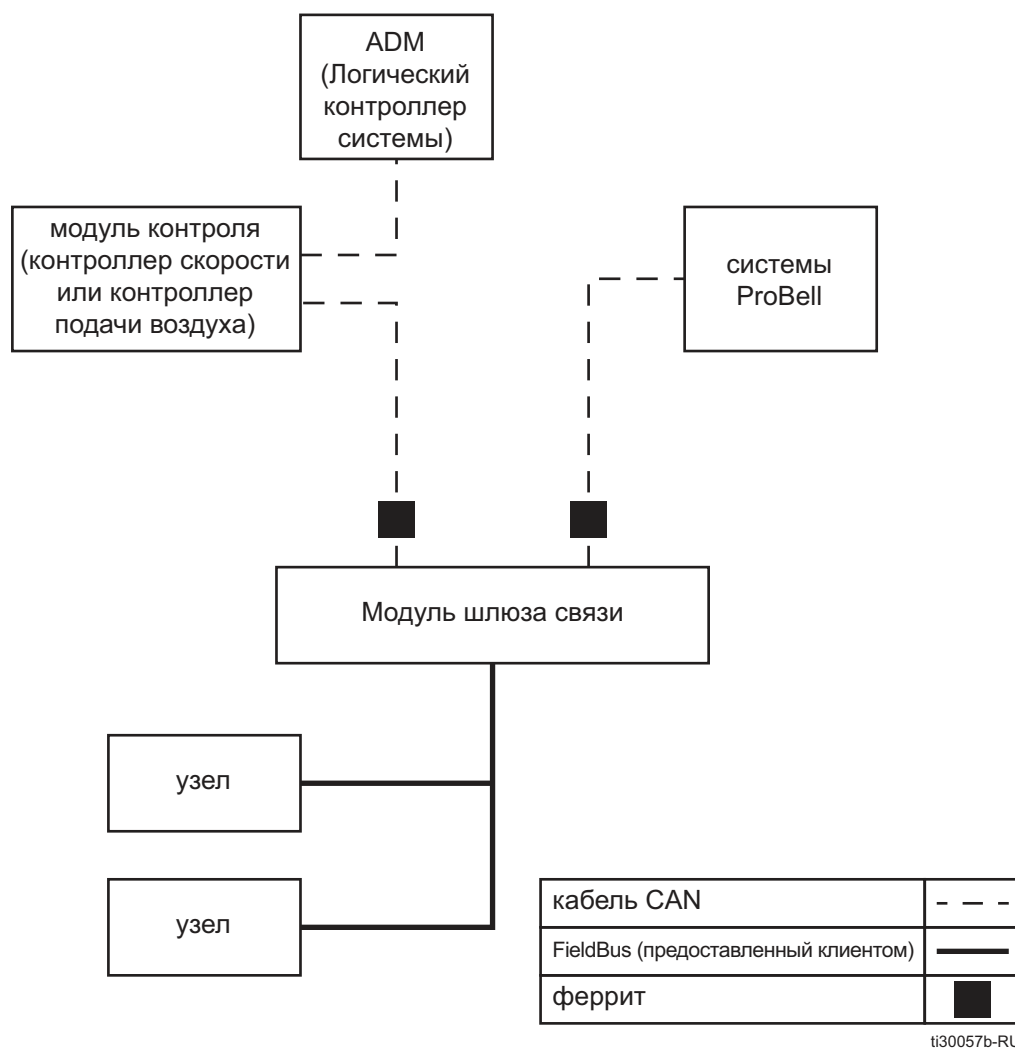
Figure 1 Схема связи между компонентами системы ProBell
