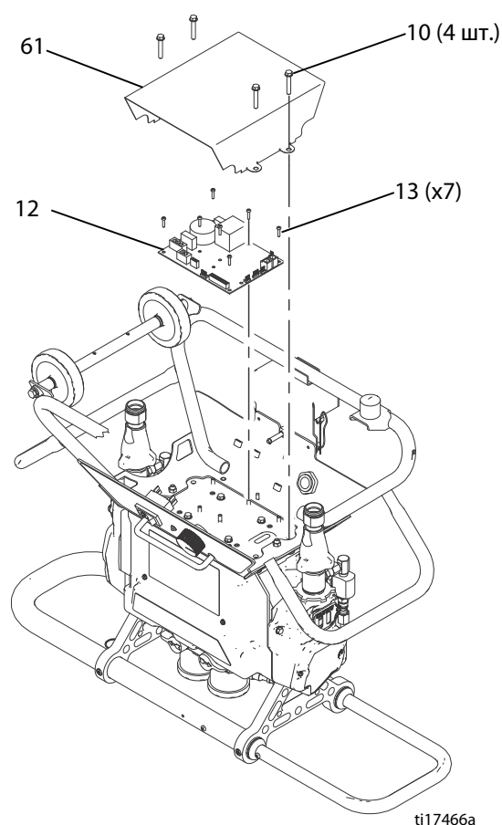
Рис. 55: Снятие платы управления
