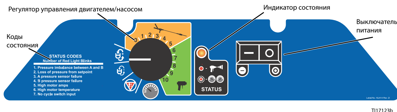
Рис. 2: Органы управления и индикаторы
