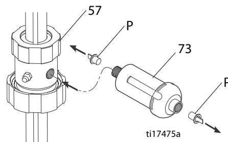
Рис. 6: Установка влагопоглотителя
