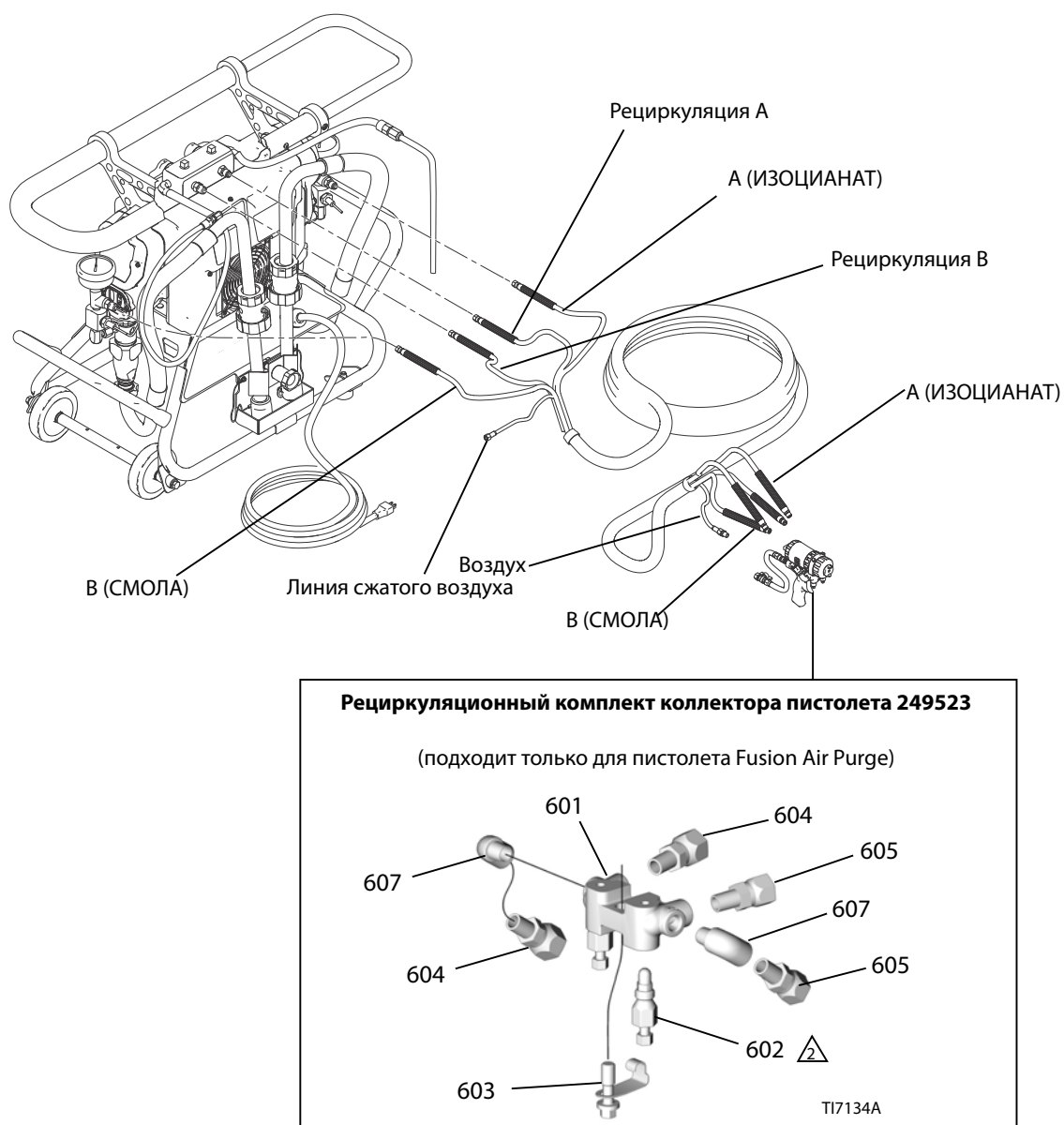
Рис. 10: Подключение шлангов и воздуха – шланговый рециркуляционный комплект 24М654
